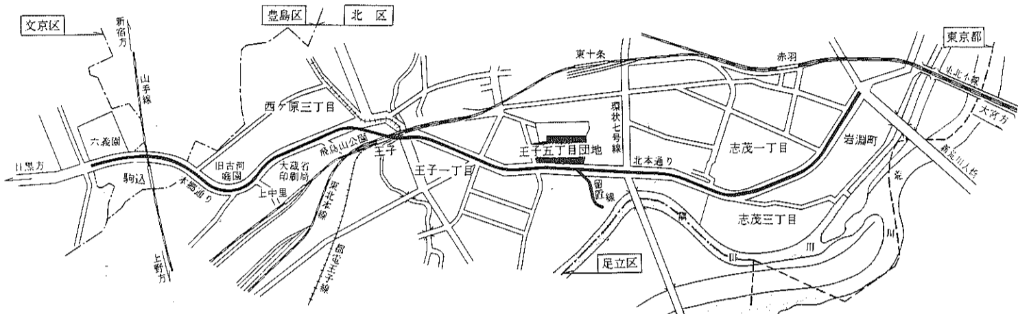
7号線 第一期 駒込・岩淵町間建設計画概要図
